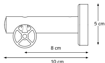
CRS Wandsteun, enkel 8 cm Ø 20 en 28 mm 12 cm Ø 20 en 28 mm 16 cm Ø 20 en 28 mm
